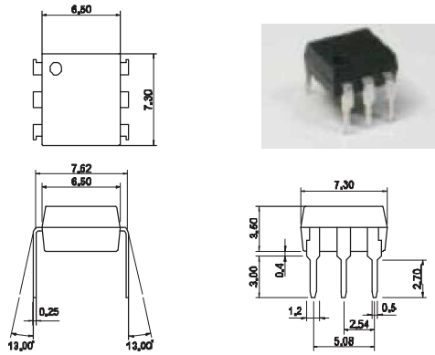
Fig.4 : 6-pln DIP type
