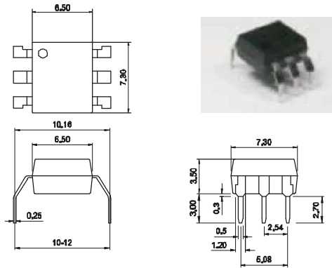
Fig.6 : 6-pln G type
