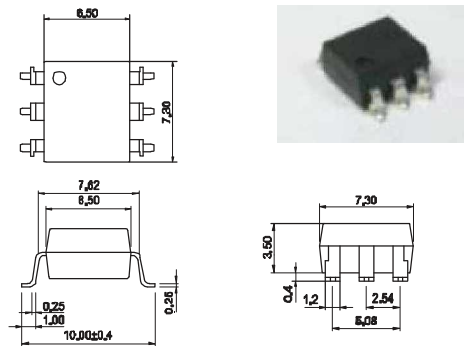
Fig.5 : 6-pln SMD type
